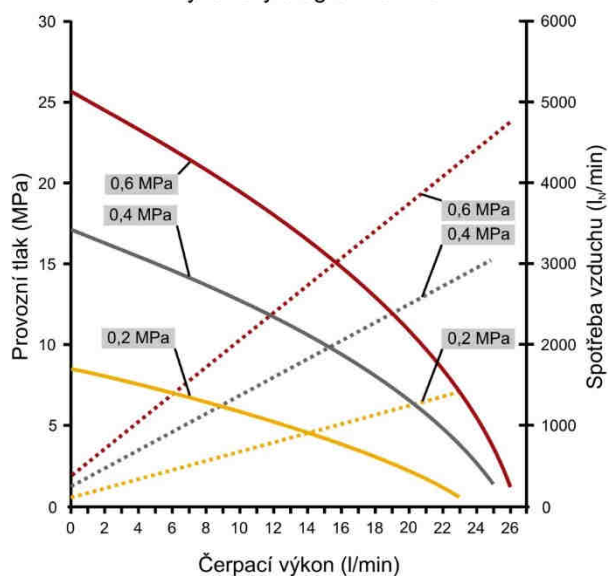
Výkonový diagram GX 45
