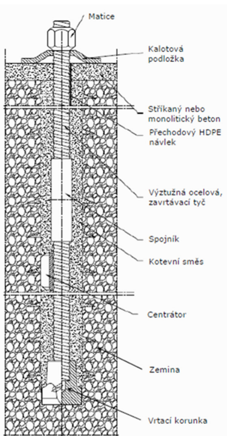
Svorník / Hřebík
