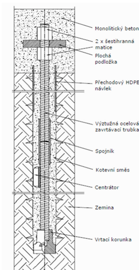
Mikropilota
